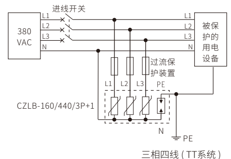
三相四线 (TT系统)
