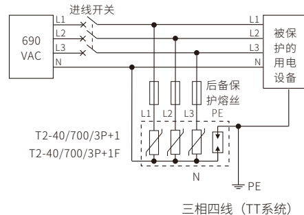
三相四线 (TT系统)
