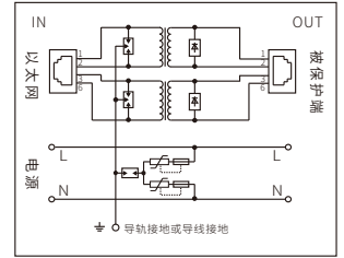
iFL-RJ45-2 百兆、220VAC电源组合
