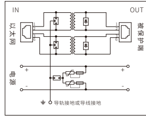
iFL-RJ45-2 百兆、24VDC电源组合
