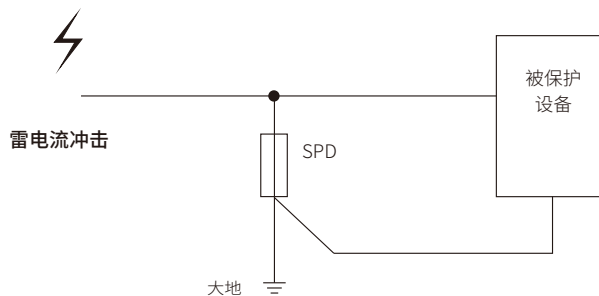
雷电流经过时，SPD瞬时对地短路，将雷电流泄放到大地
