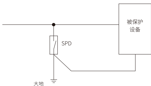
无雷电流时，SPD对地保持开路
